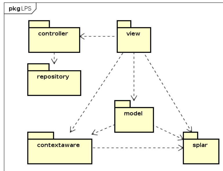
Figura 21 – Diagrama de pacotes.
