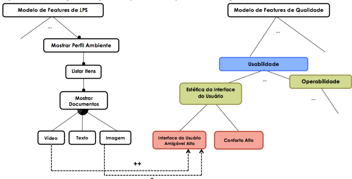
Figura 17 – Exemplo da representação de restrições de interdependências entre Features e PNFs
