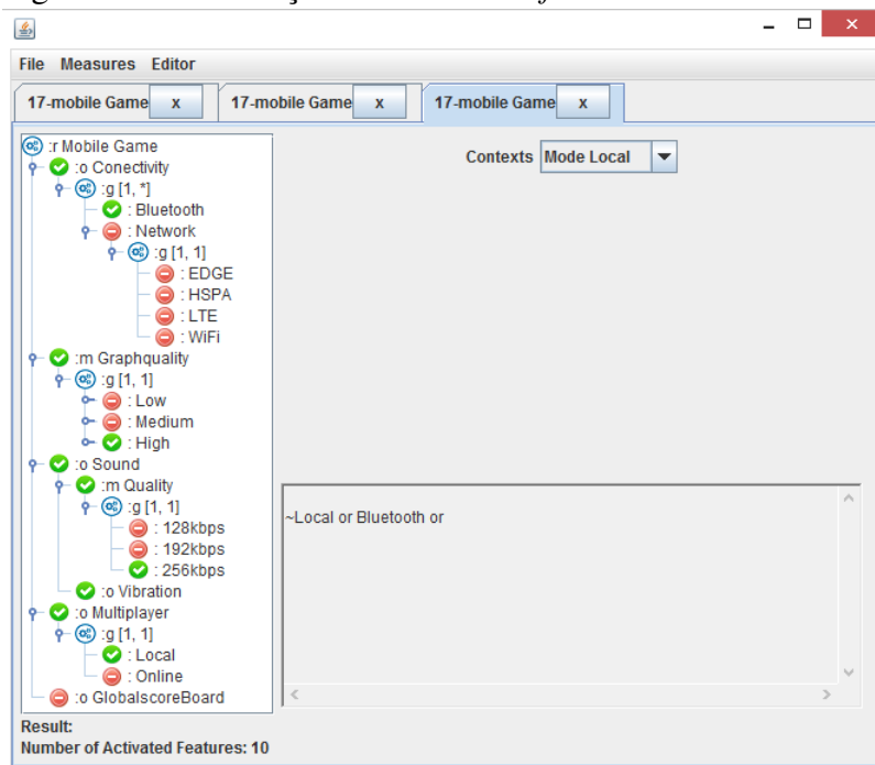
Figura 9 – Visualização do modelo de features .
