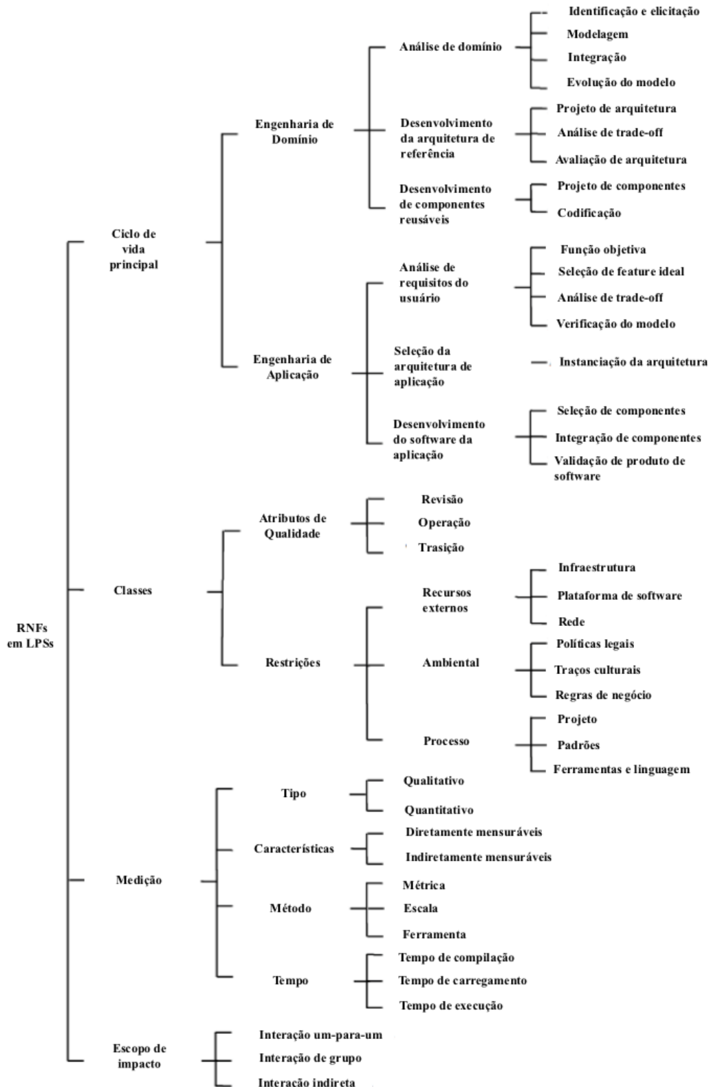
Figura 2 – Taxonomia para RNFs em linhas de produtos de software.
