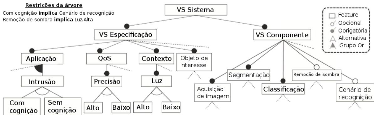
Figura 7 – Modelo de features com notação da abordagem (FM-QC).
