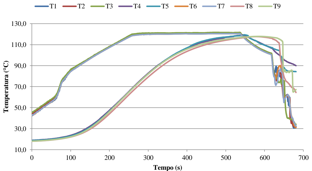
Gráfico 1 - Processamento térmico da sopa de vegetais e carne à base de maracujá silvestre (Repetição 1)
