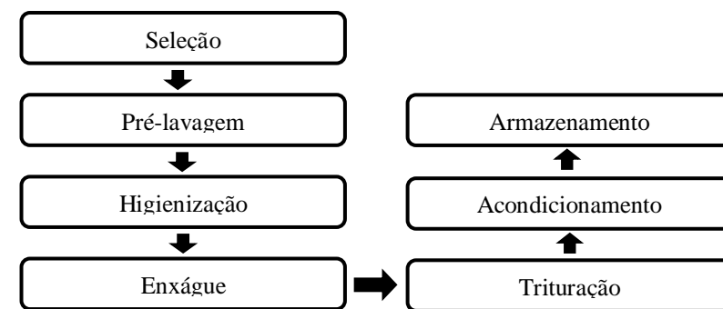
Figura 2 - Fluxograma de processamento da massa base de maracujá silvestre ( P. tenuifila Killip)
