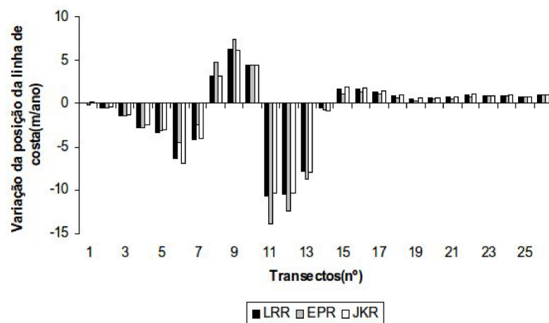
Figura 5 – Taxas de variação da margem esquerda do Jaguaribe, iniciando-se na desembocadura até o estuário inferior (valores negativos indicam erosão).
